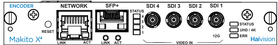
Makito X4 Encoder
